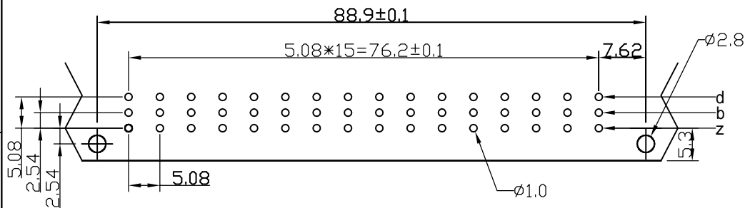
P.C.Board Layout
