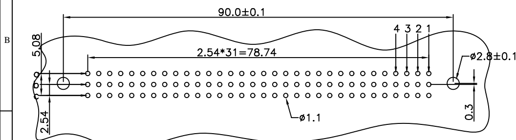
P.C.Board Layout
